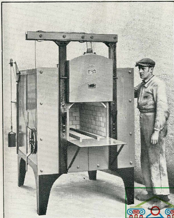
Four à tremper, recuire et cémenter
